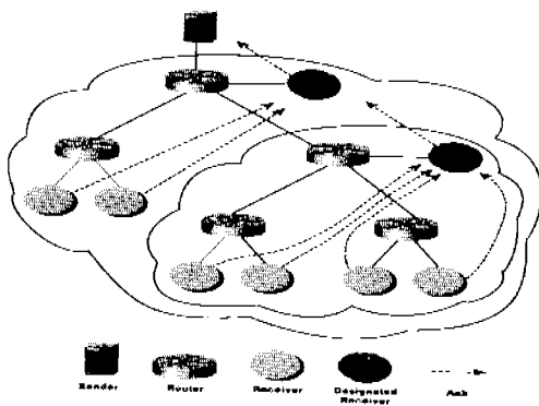
그림 4. 트리 기반 신뢰전송 프로토콜
