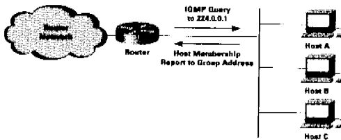
그림 2. IGMP 동작원리
